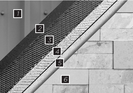
FIG. 5. PAROI MÉTALLIQUE
