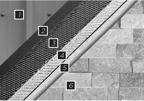
FIG. 5. PAROI MÉTALLIQUE
